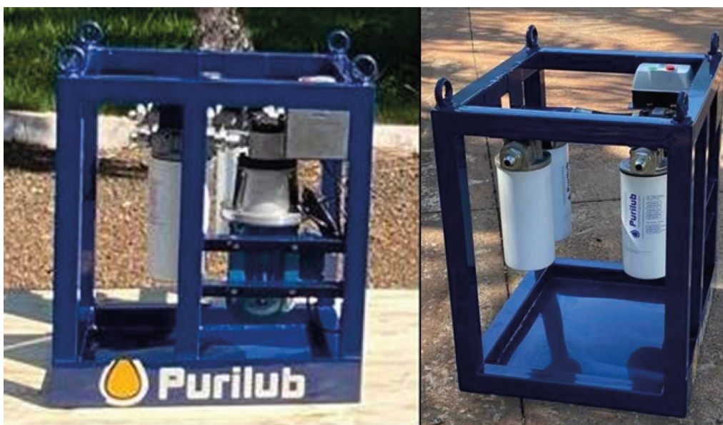
Figura 1 - Unidade para purificação de gear box de aerogerador.
